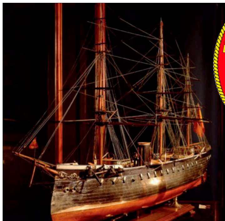
Modelo original de la fragata «Numancia». ARMADA ESPAÑOLA
